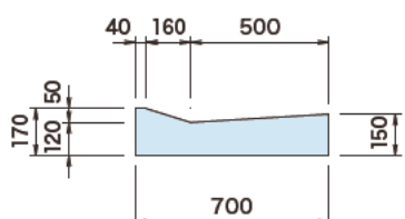
●断面図
