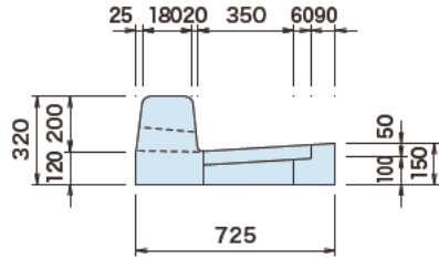
●断面図
