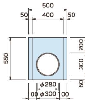
●側面図
