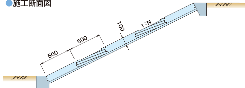
● 施工断面図
