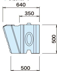
寸法表
