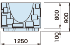
●施工断面図(標準)
