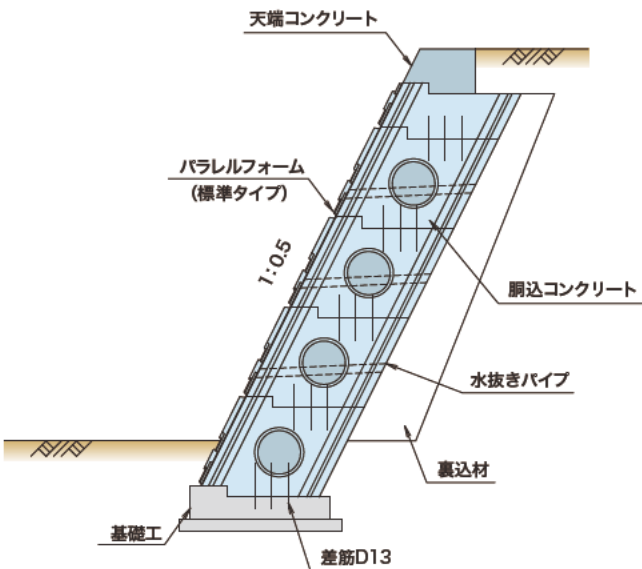
●施工断面図(標準)
