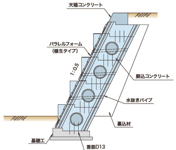
●施工断面図(植生)
