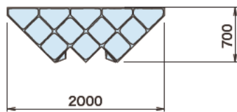
●正面図
