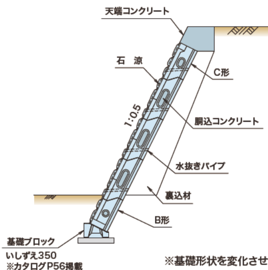
●施工断面図 (5分勾配の場合)
