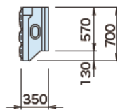
●側面図
