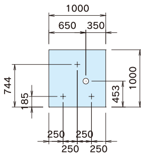
●B・D型表面図
