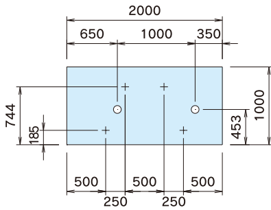
●A・C型表面図
