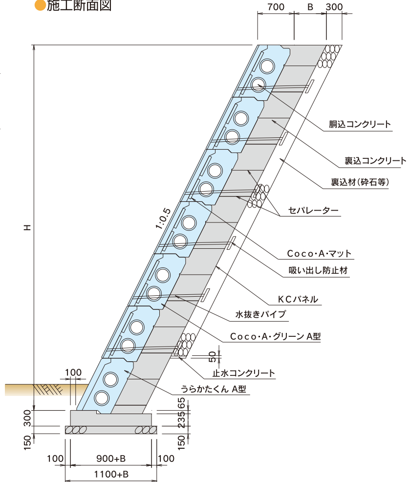
●施工断面図
