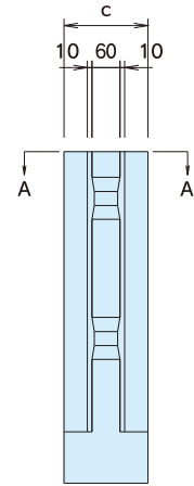
●側面図
