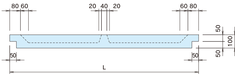
● 側面図
