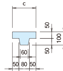
●A-A' 断面図
