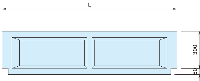
● 側面図
