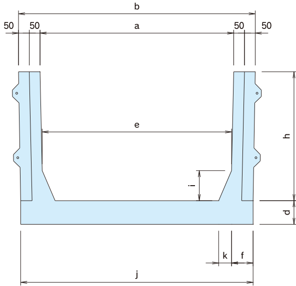
●断面図
