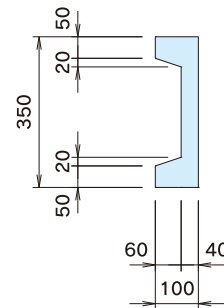
● 断面図
