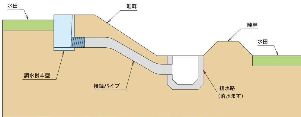
● 施工概略図
