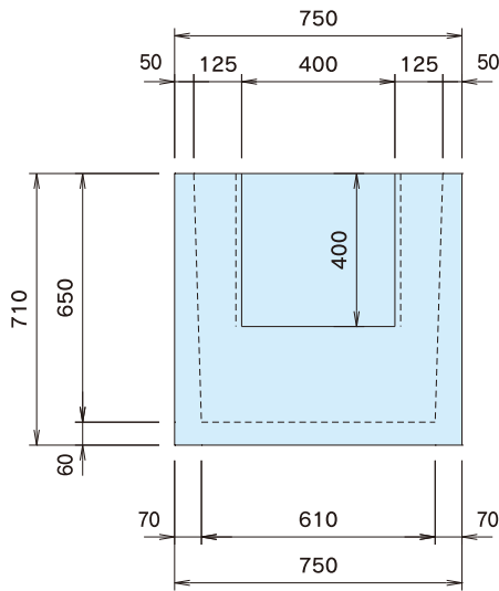
● 側面図 (650型)
