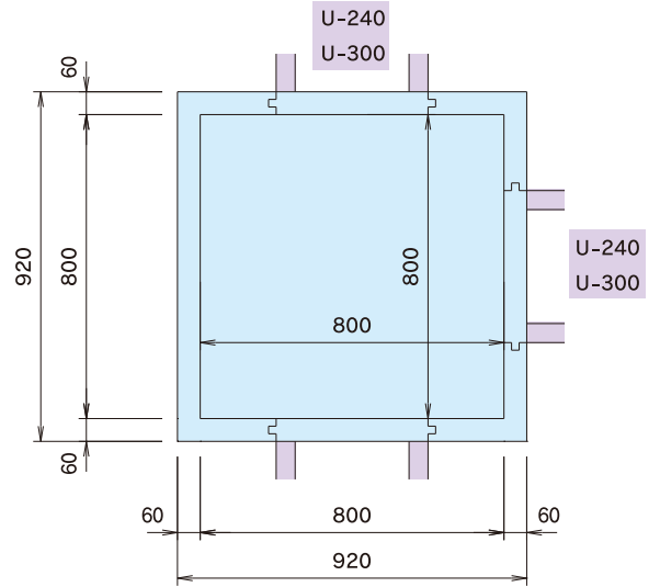
● 平面図 (800型)
