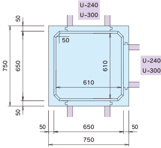
● 平面図 (650型)
