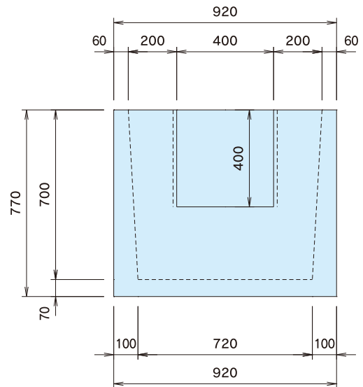
● 側面図 (800型)
