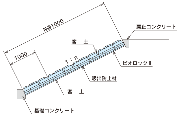
● 標準施工図
