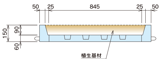
● A-A'断面図
