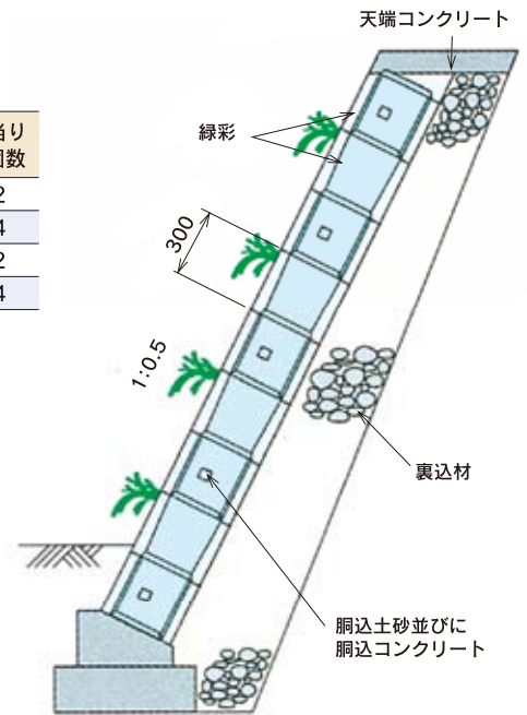
●施工断面図
