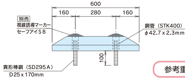
●正面図
