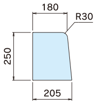
●断面図
