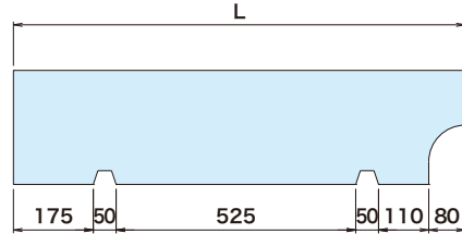
●正面図
